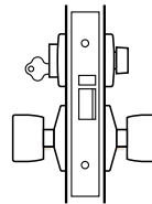
Antilockout Entry Door Lock
